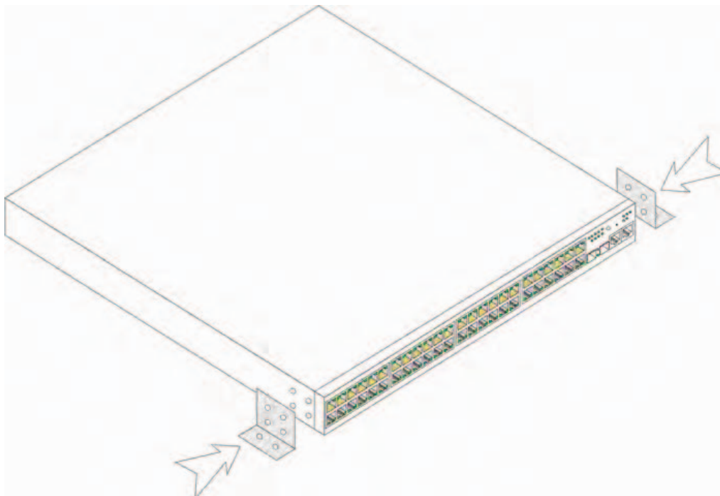
Obr. 1-2. Instalace držáku při montáži na zed'
